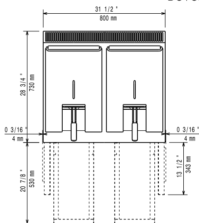
Boven aanzicht
